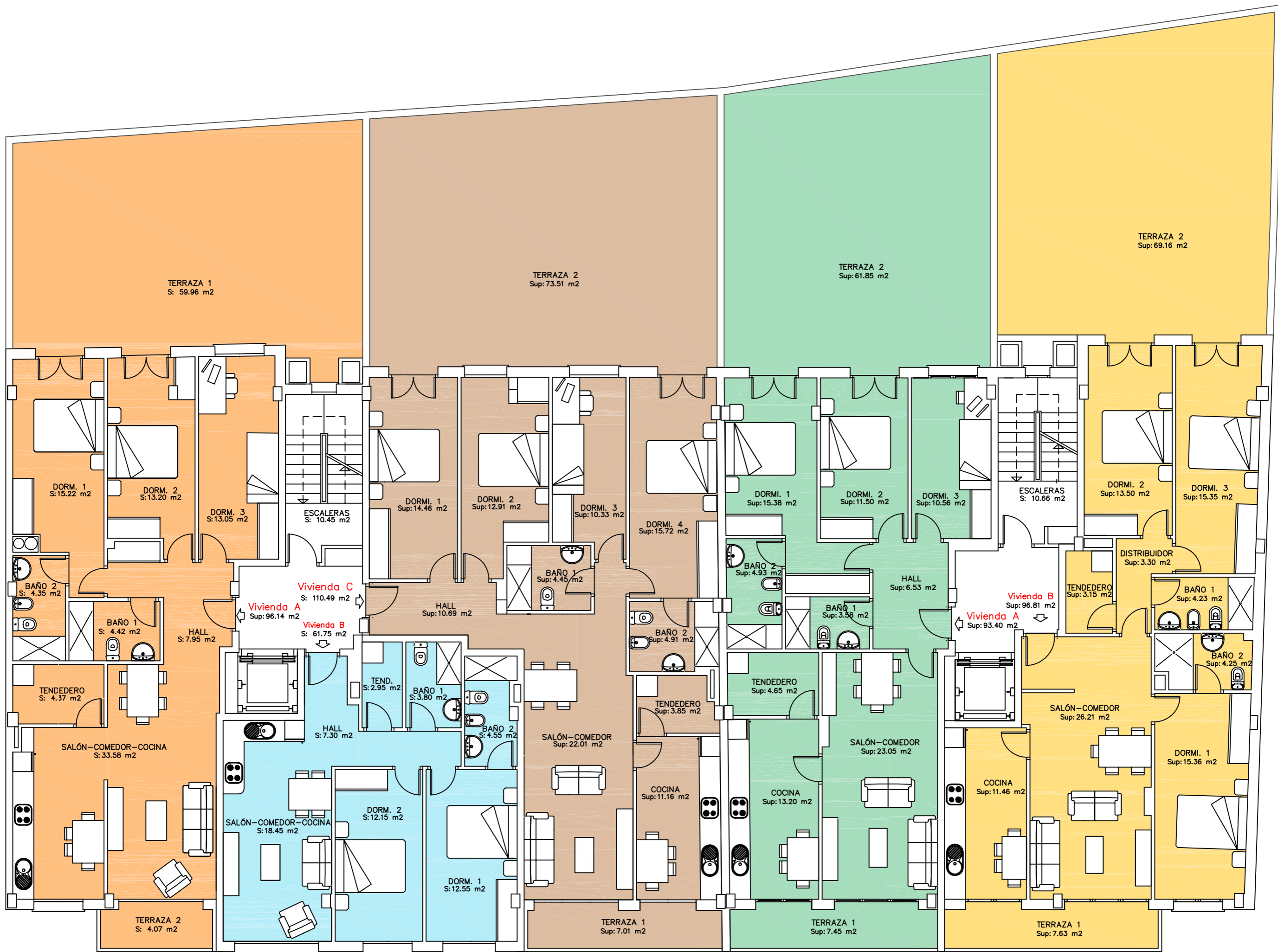
PLANTA TIPO
